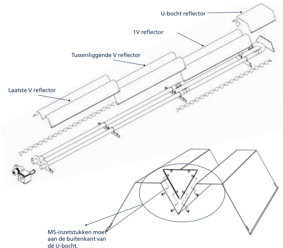
Figuur 28. Reflectoren
