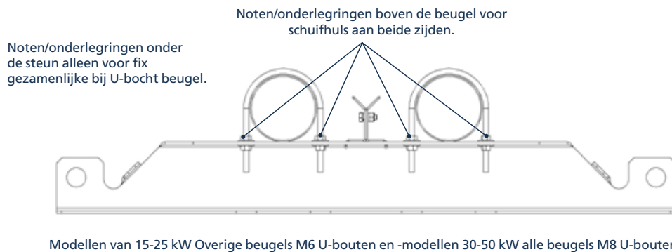
Figuur 26. U-bout op de U-vormige buis kachel ophangbeugels
