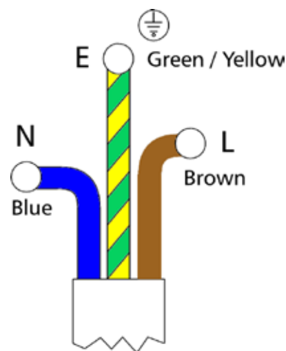
Figuur 14. Enkelfasig bedrading
