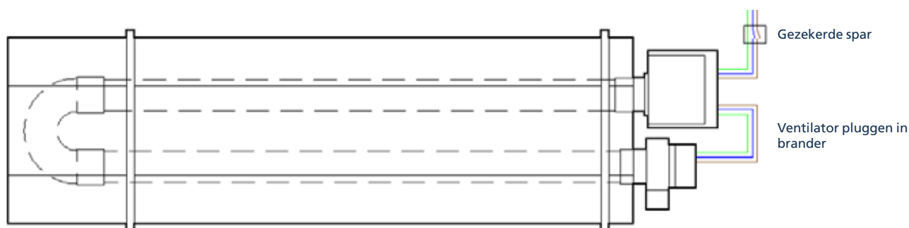
Figuur 15. Typische VSUTE bedradingsaansluitingen
