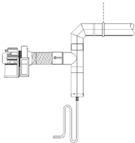
Figuur 6.7 Typische low fan regeling
