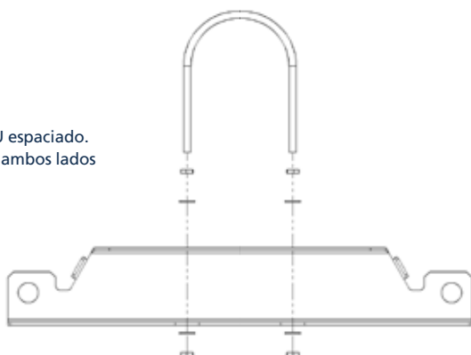
Ilustración 26.5 Fijación de pernos en U en los soportes de suspensión del calefactor de tubo en U
