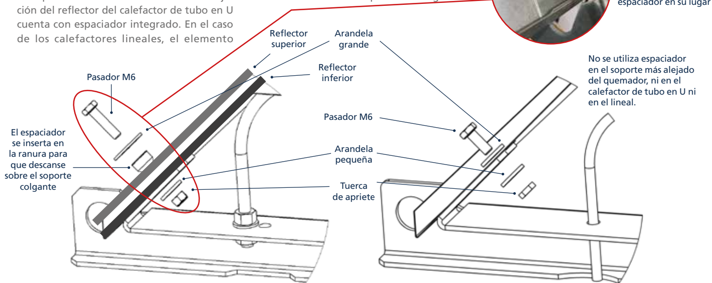
Ilustración 31. Reflector en V de tubo en U intermedio
