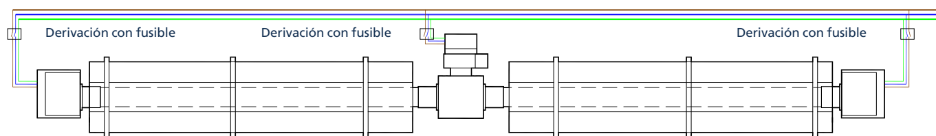
Ilustración 15.2 Conexiones típicas de cableado de VSDLE unitario
