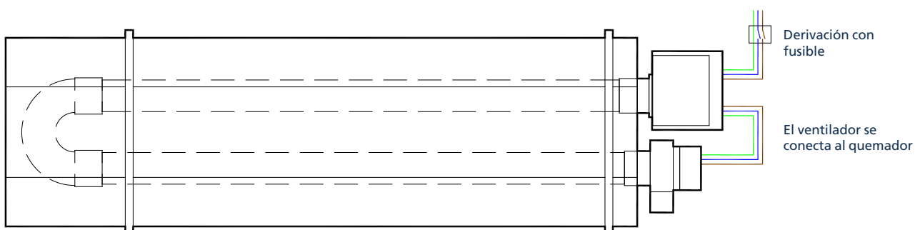
Ilustración 15. Conexiones típicas de cableado de VSUTE
