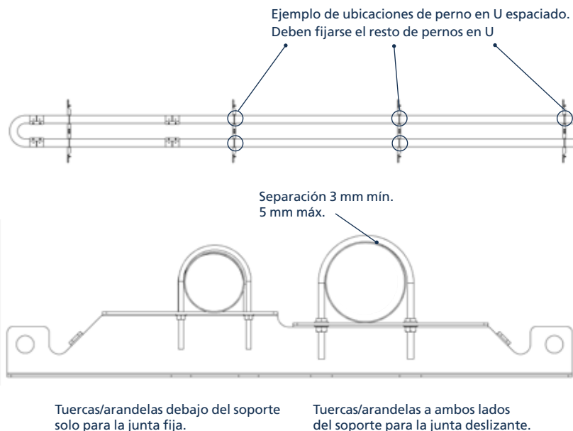
Ilustración 26.3 Fijación de pernos en U en los soportes de suspensión del calefactor de tubo en U
