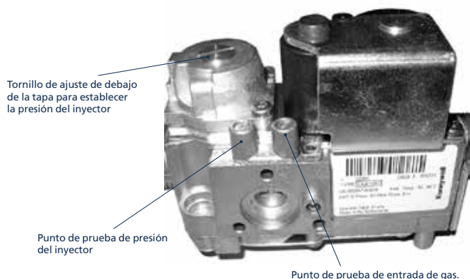
Ilustración 53. Honeywell serie VK4105
