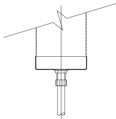
Ilustración 6.1 Disposición de la trampa colectora de condensado
