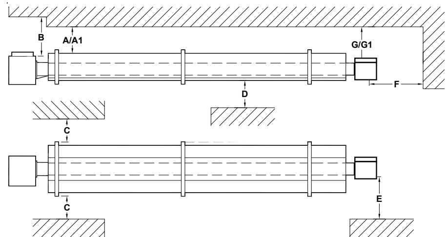
Ilustración 10. Esquema que ilustra la distancia a los combustibles (lineal)
