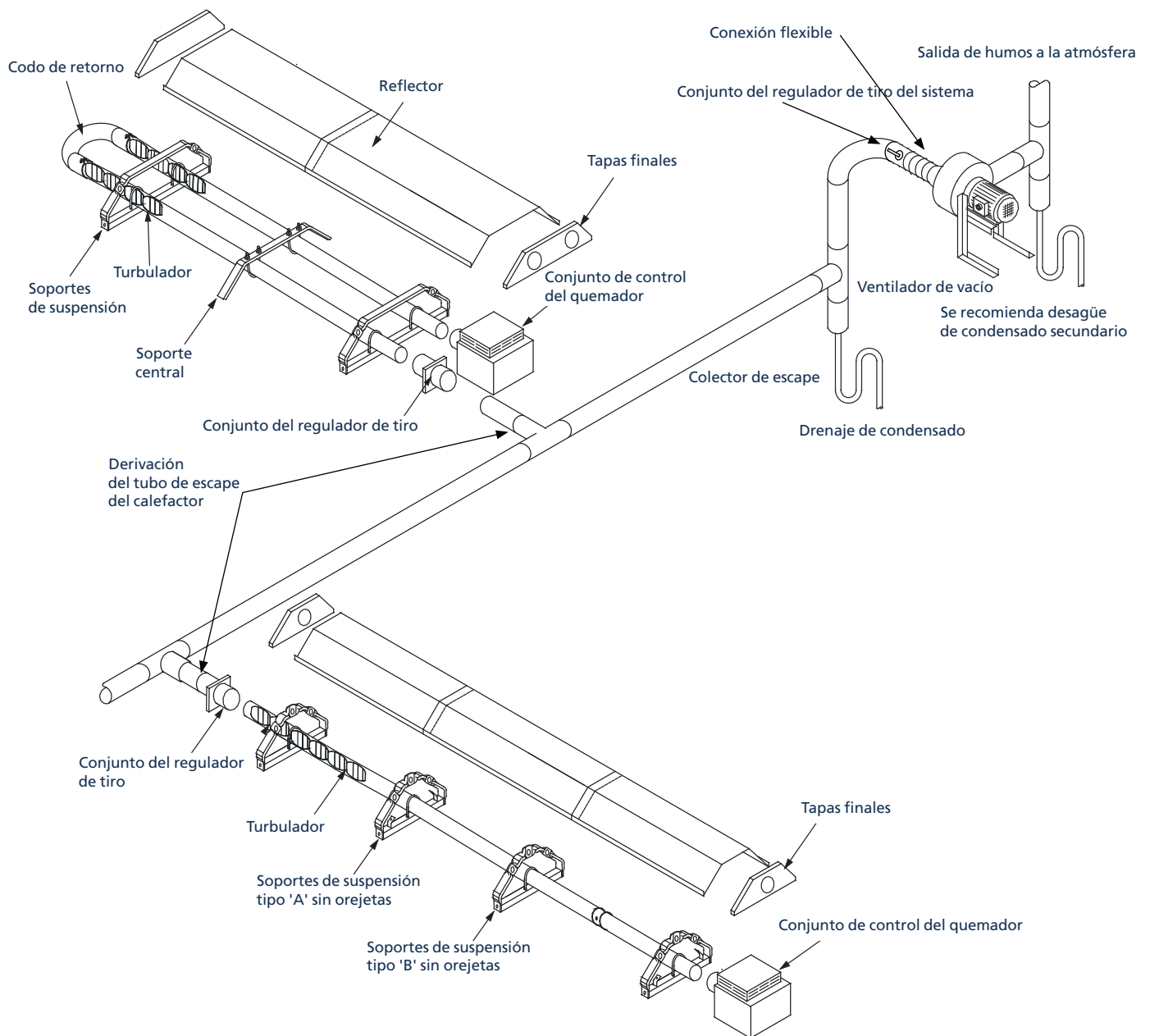
Ilustración 8. Instalación en espiga
