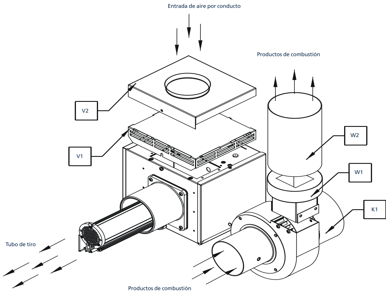
Ilustración 18. Opción 1. Acoplamiento del sistema de salida de humos a quemadores inducidos (VSUTE)
