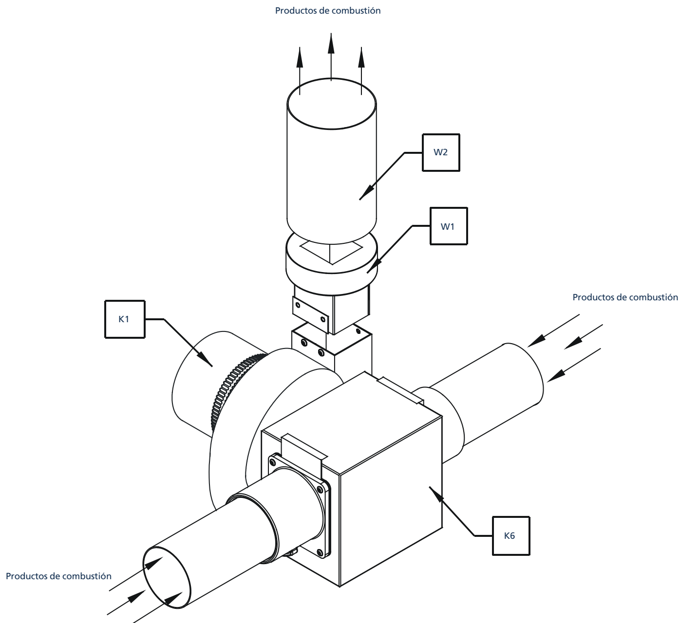
Ilustración 19. Opción 2. Acoplamiento del sistema de salida de humos a quemadores inducidos (VSDLE)
