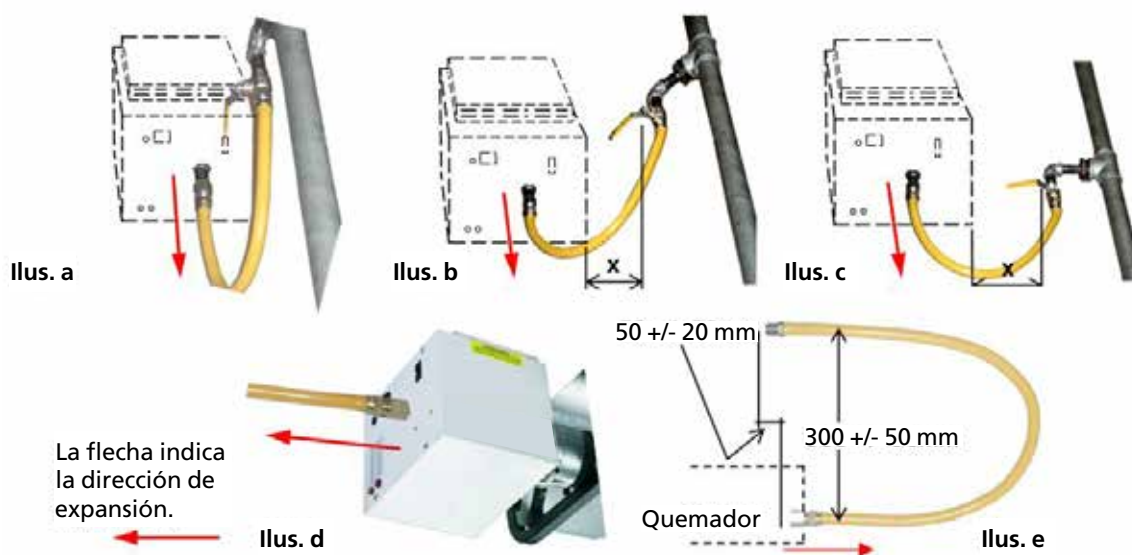
Ilustración 11. Instalación correcta del tubo de gas flexible
