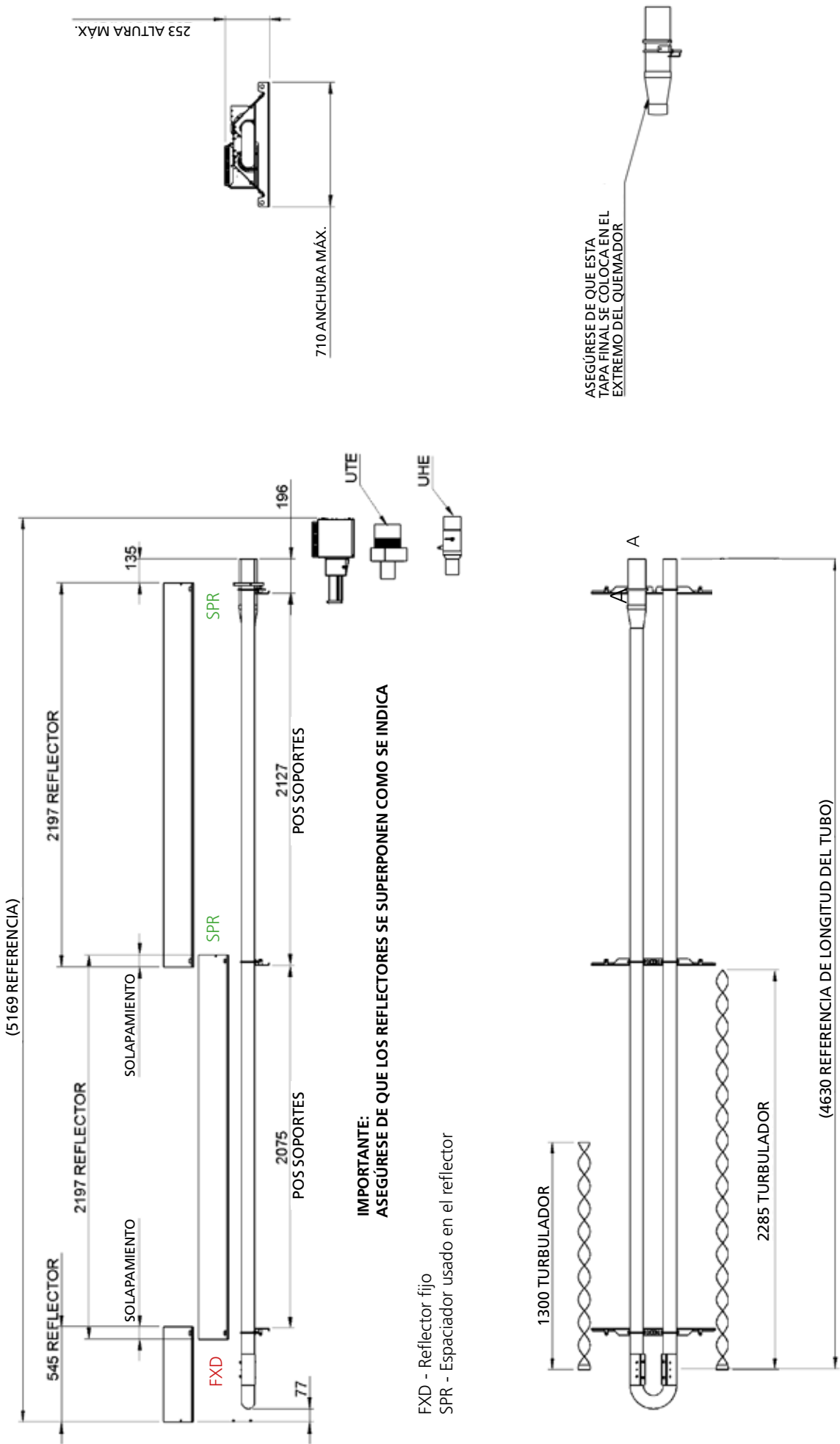
Ilustración 42. Conjunto del calefactor Vision: Modelos VSUTE/VSUHE 20/25 kW. Diá. nom. 76 mm (3 pulg.)
