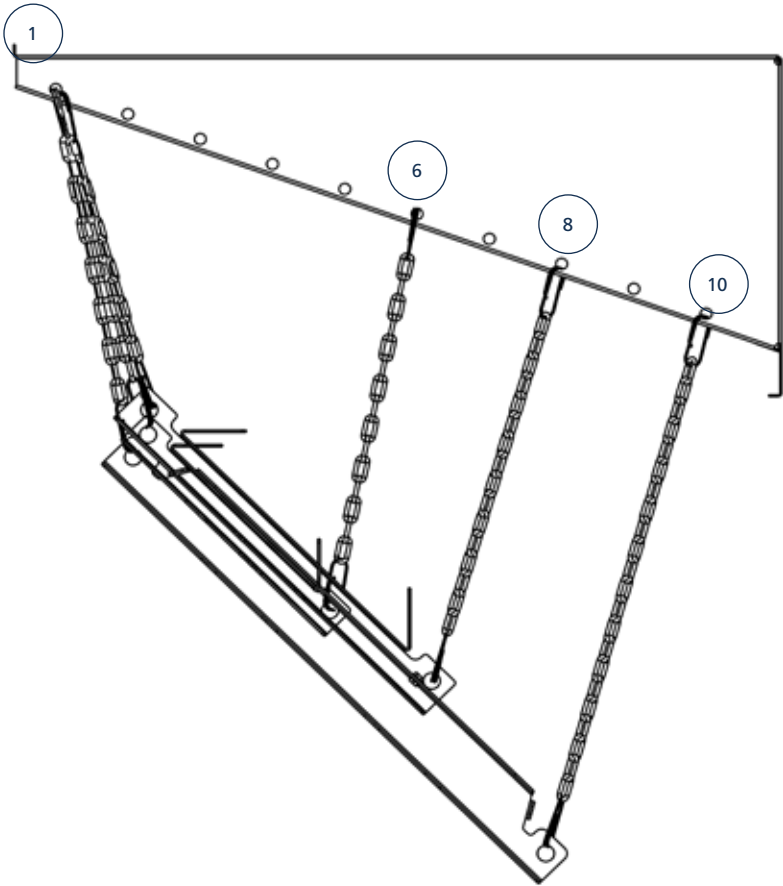
Ilustración 1. Montaje en ángulo utilizando el soporte de montaje en pared
