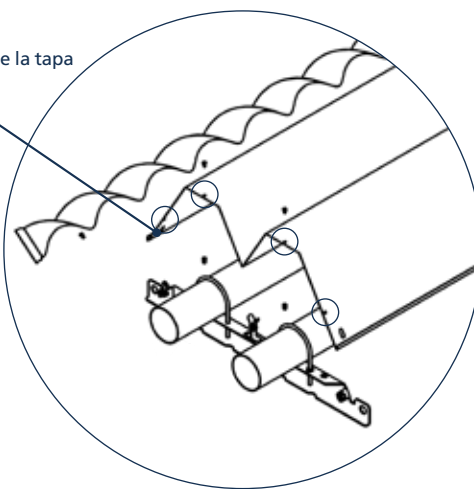
Ilustración 29. Reflector en V de tubo en U final
