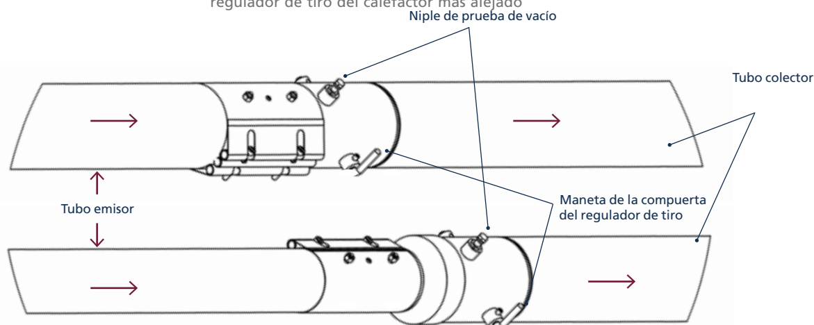
Ilustración 51. Conjunto del regulador de tiro en espiga
