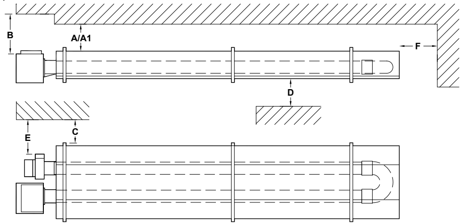
Ilustración 9. Esquema que ilustra la distancia a los combustibles (tubo en U)
