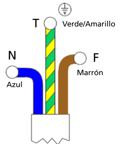
Ilustración 14. Cableado monofásico
