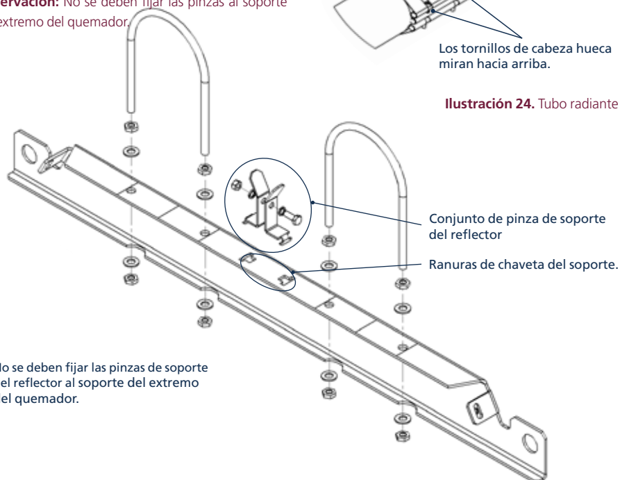
Ilustración 25. Soporte de reflector
