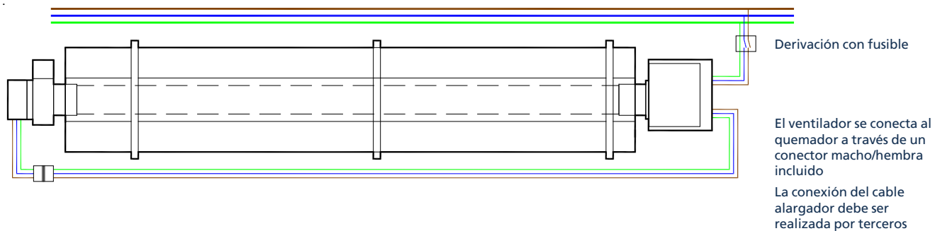
Ilustración 15.1 Conexiones típicas de cableado de VSLIE
