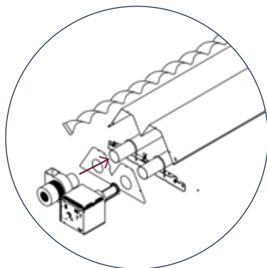
Ilustración 36. Conjunto del ventilador del modelo de tubo en U
