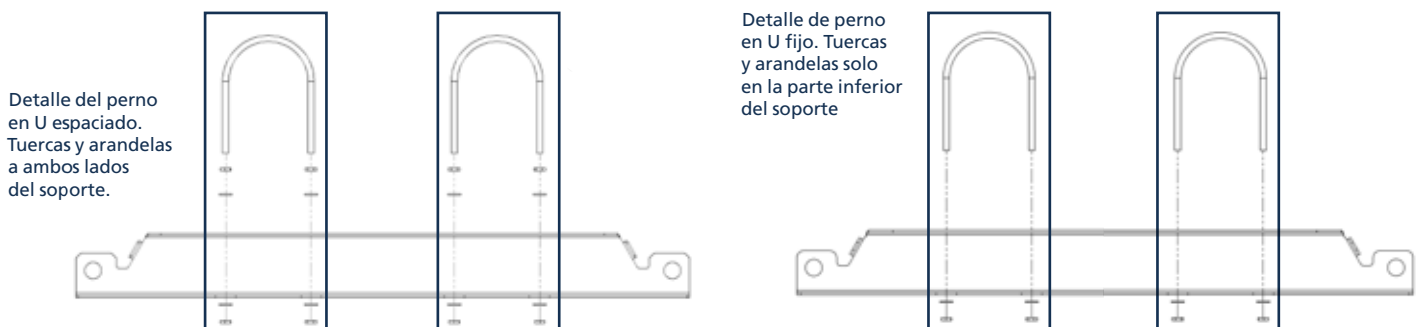
Ilustración 26.2 Fijación de pernos en U en los soportes de suspensión del calefactor de tubo en U
