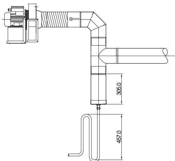
Ilustración 6. Disposición de la trampa de condensado
