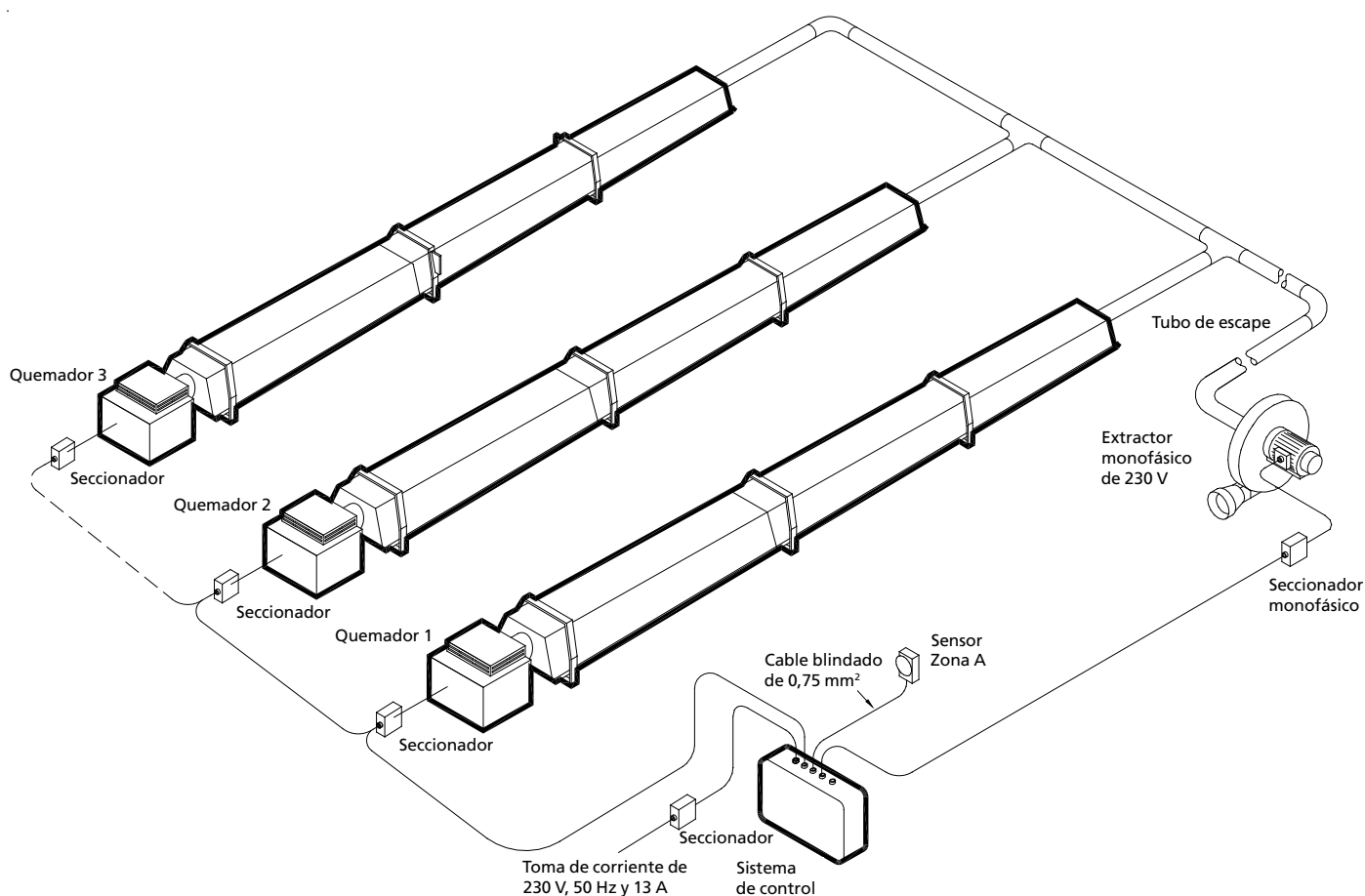
Ilustración 16. Conexiones típicas de cableado de VSLHE unitario
