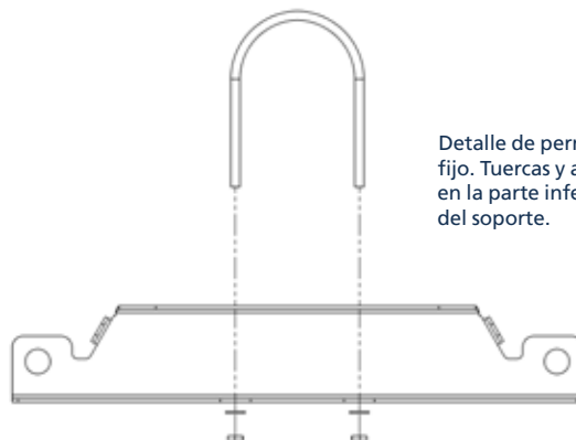
Ilustración 26.5 Fijación de pernos en U en los soportes de suspensión del calefactor de tubo en U
