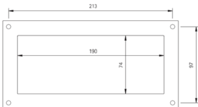
Ilustración 6.2 Dimensiones de la salida del ventilador tipo 'O'
