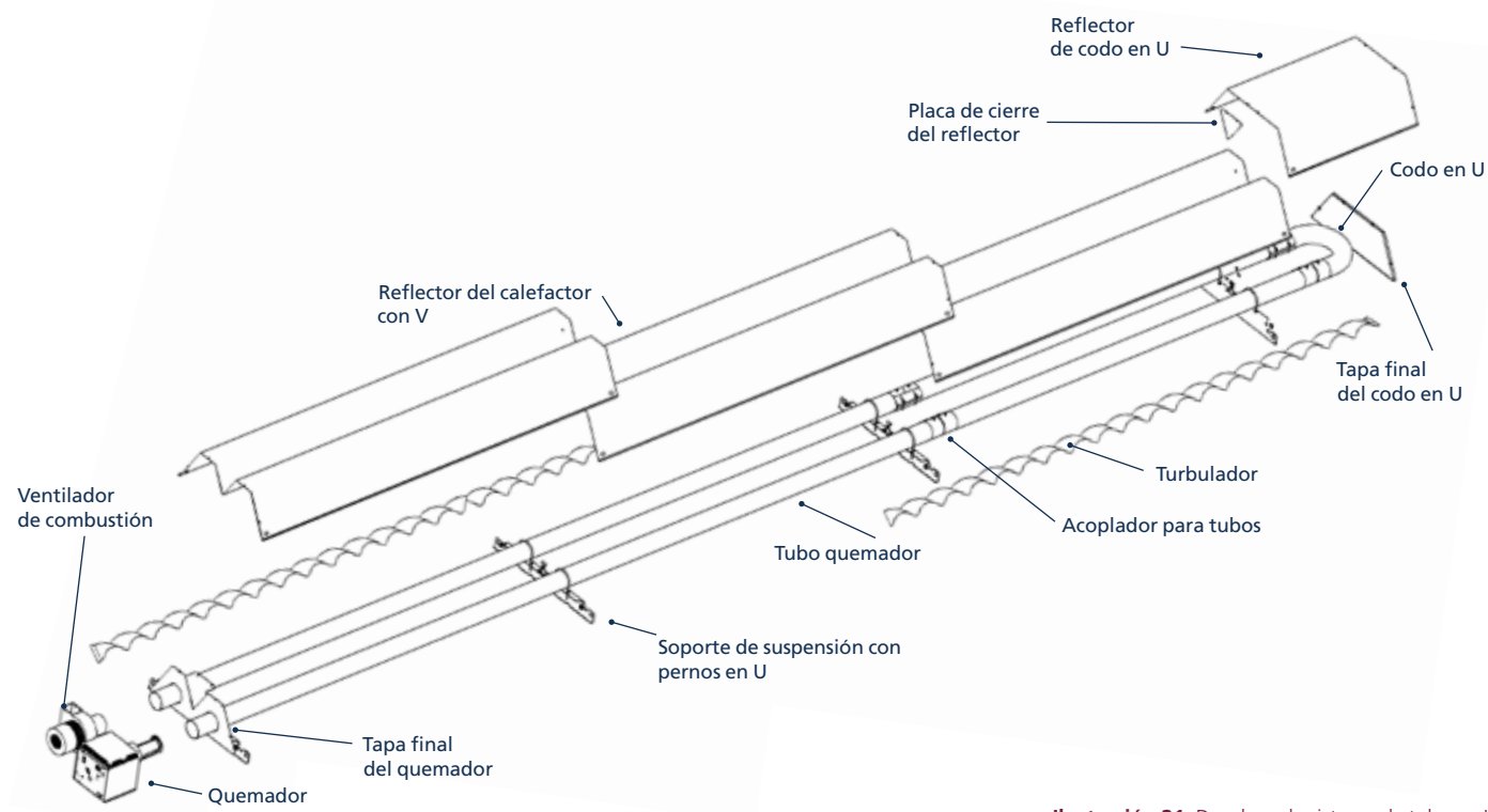
Ilustración 21. Desglose de sistema de tubo en U
