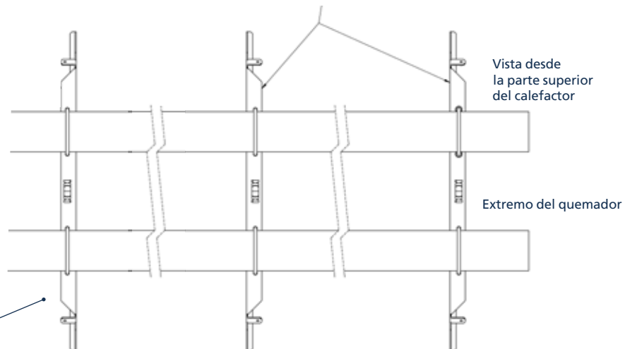
Ilustración 26.1 Fijación de pernos en U en los soportes de suspensión del calefactor de tubo en U
