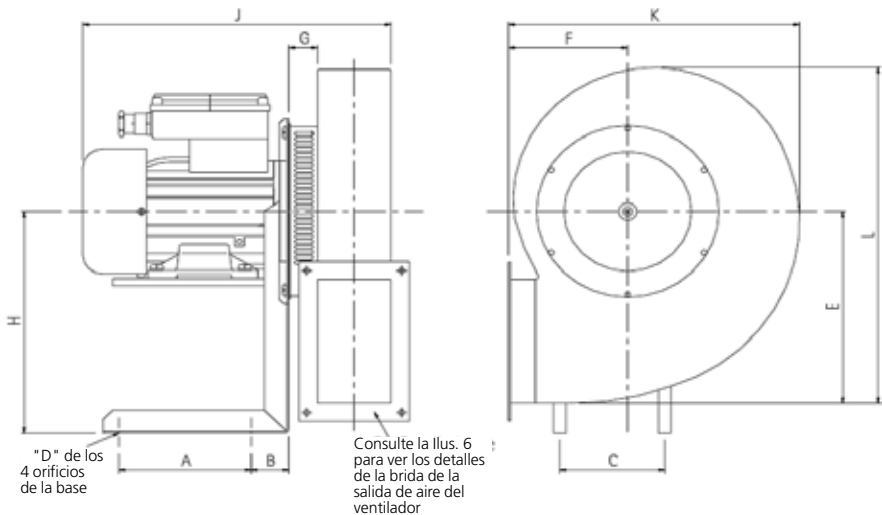
Ilustración 7. Información de montaje del ventilador de vacío (ilustración del ventilador tipo 'O')
