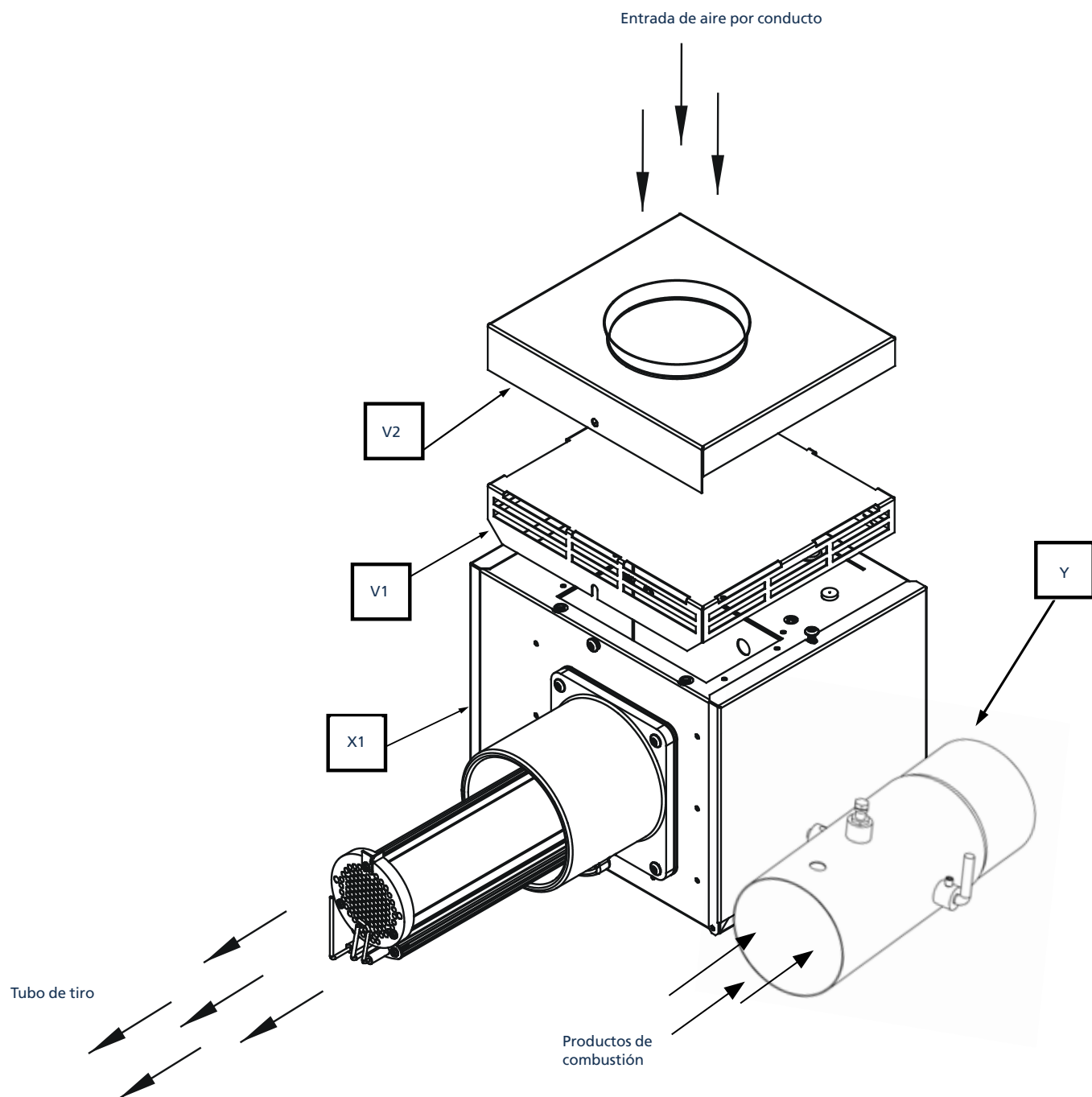
Ilustración 20. Opción 3. Acoplamiento del sistema de salida de humos a quemadores inducidos (VSLHE)
