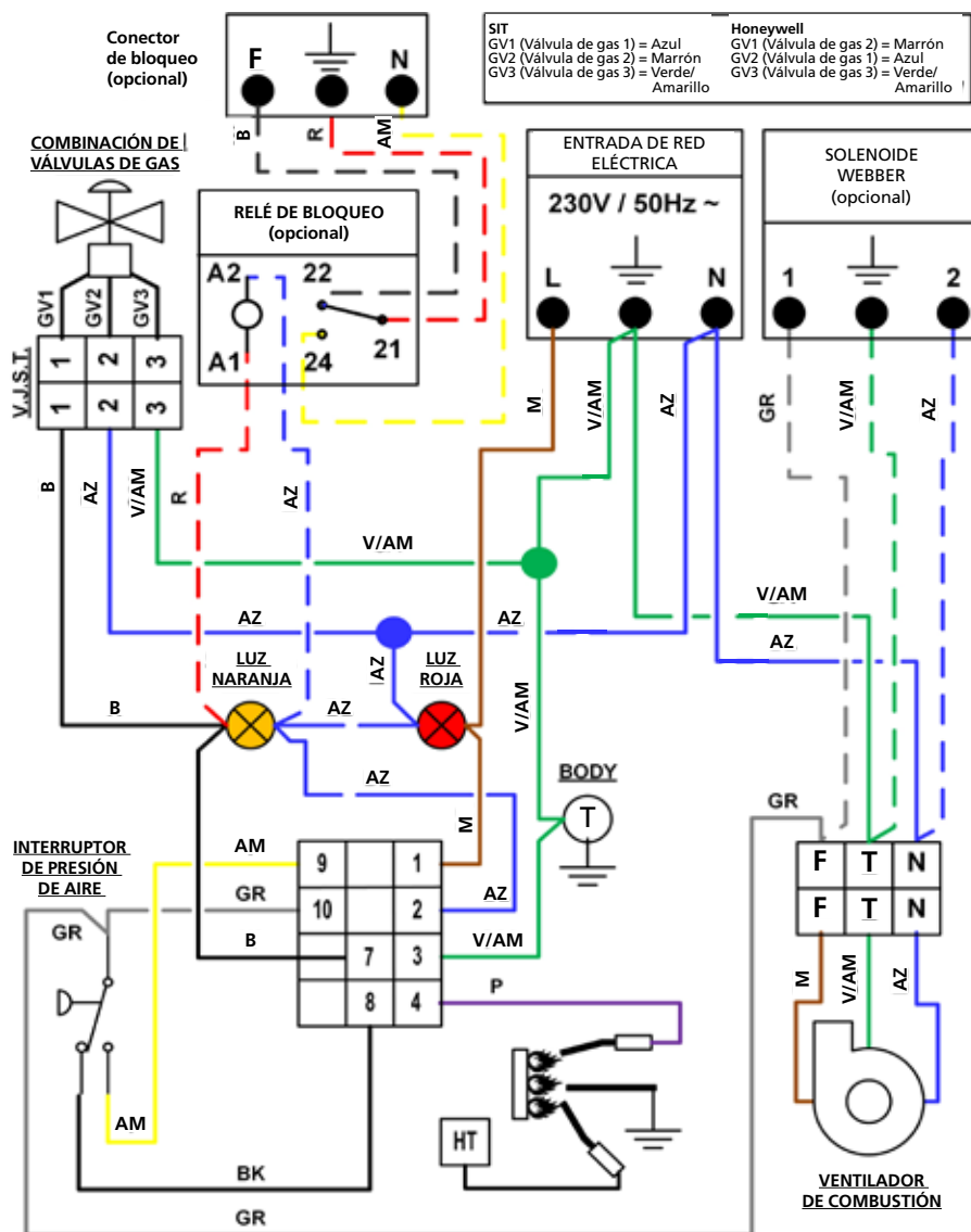
Ilustración 17. Esquema de cableado del quemador interno de VS
