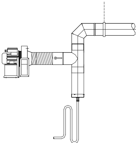
Figure 6.7 Disposición típica de ventilador bajo
