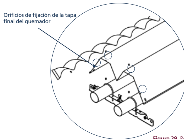
Figure 29. Reflector en V de tubo en U final
