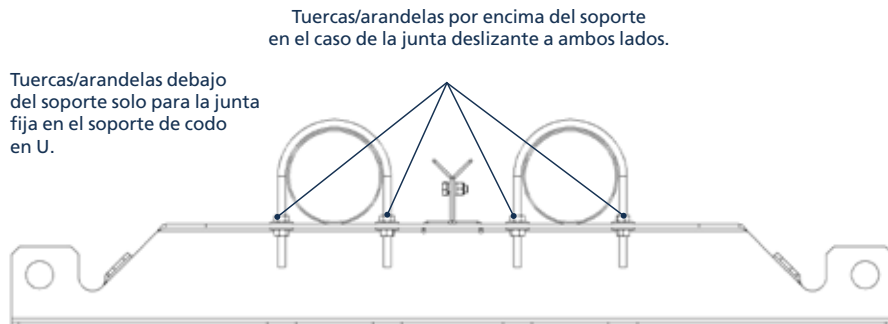
Pernos en U M6 de los soportes restantes de los modelos 15-25 kW y pernos en U M8 de todos los soportes de los modelos de 35-50 kW.
