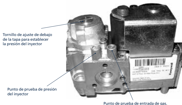
Figure 53. Honeywell serie VK4105
