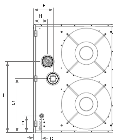
Achteraanzicht Photon 120
