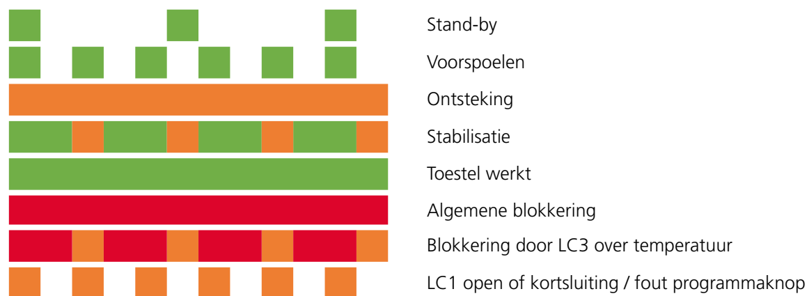
Figuur 9 LED-status
