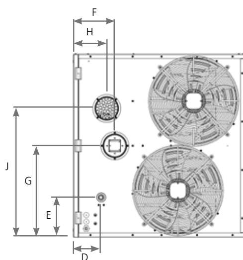
Achteraanzicht Photon 100
