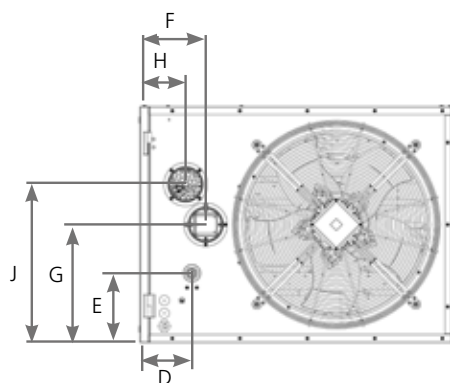
Achteraanzicht Photon 10-70
