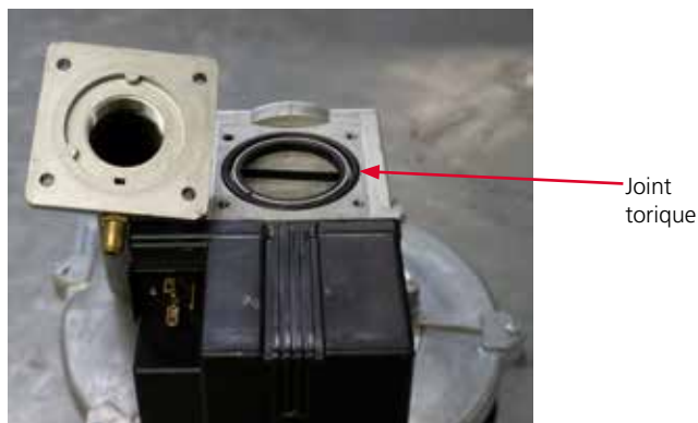
Montage de la bride d'entrée de la vanne de gaz du Photon 120
