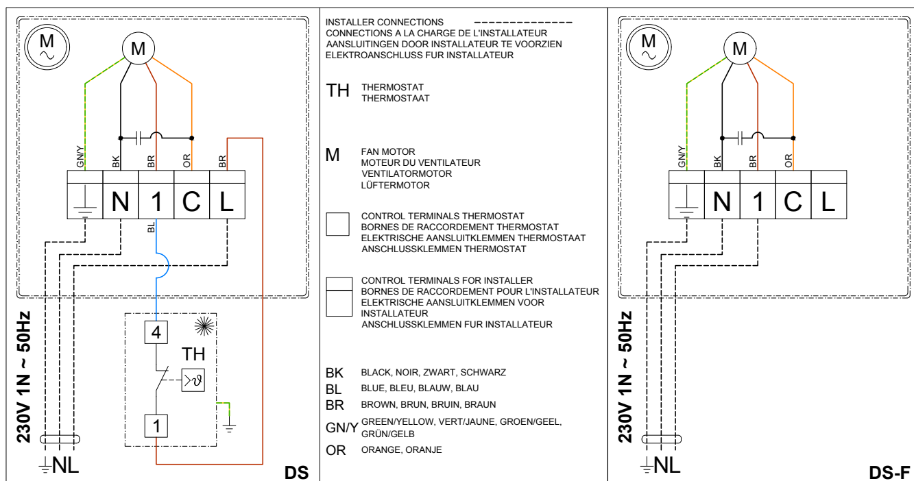
Abbildung 3 Interner Schaltplan
