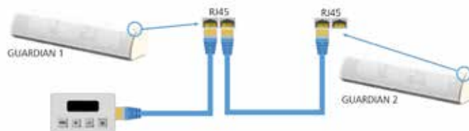
Figura 25 Cableado de 2 o más cortinas de aire en red.
