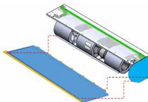
Figura 11 Panel de acceso inferior GS
