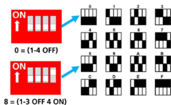
Figura 24 Números de dirección de la cortina de aire
