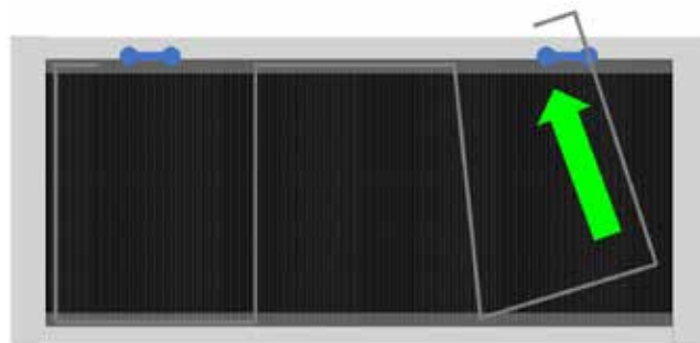
Figura 27.1 GS quitando el clip de retención de espuma de entrada
