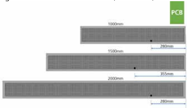
Figure 30 Position du capteur de température
