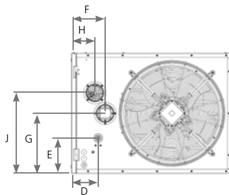
Achteraanzicht Photon 10-70
