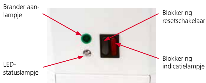
Resetschakelaar en statuslampjes
