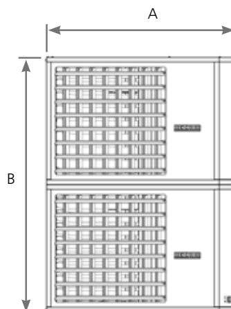
Vooraanzicht Photon 120
