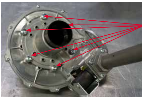
Photon 10-70 bevestigingsschroeven gaskleppen
