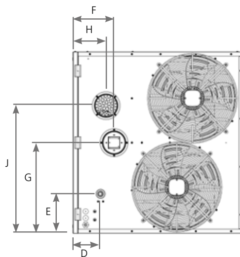
Achteraanzicht Photon 100
