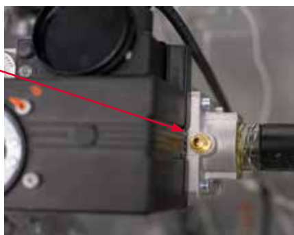
Gasdruktestpunt voor Photon 120
