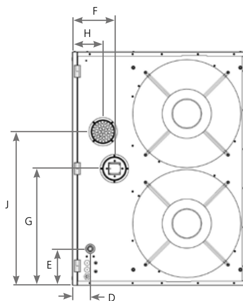
Achteraanzicht Photon 120
