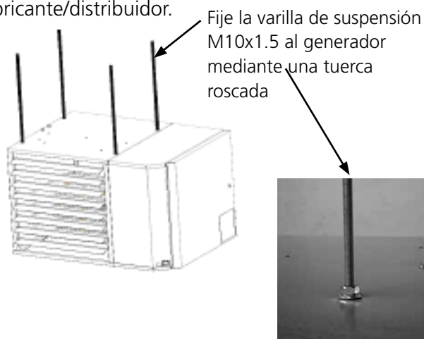
Figura 1 Suspensión del generador con varillas desde los puntos de fijación de tuerca roscada
