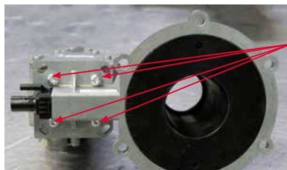
Tornillos de fijación de la válvula de gas de Photon 100
