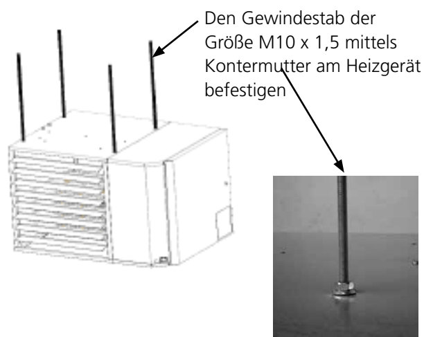
Abbildung 1 Heizgerät wird mittels in die Gewindemutterhalterungen eingeschraubten Gewindestäben abgehängt
