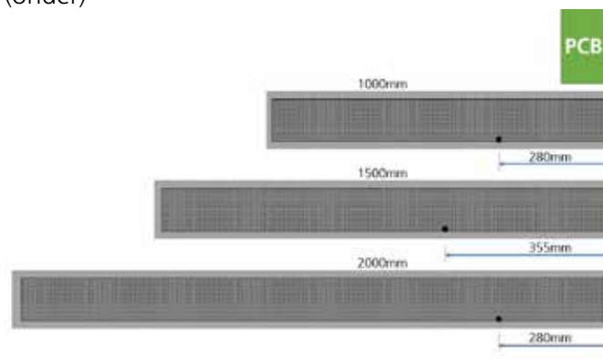
Fig 30 Temperatuursensor positie
