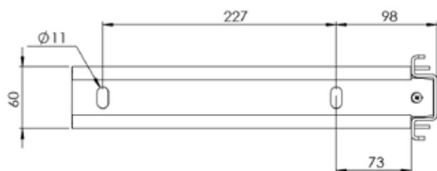
Fig 15.3 Montagebeugel bovenaanzicht
