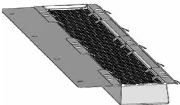
Fig 29.1 GR-honingraatkering
