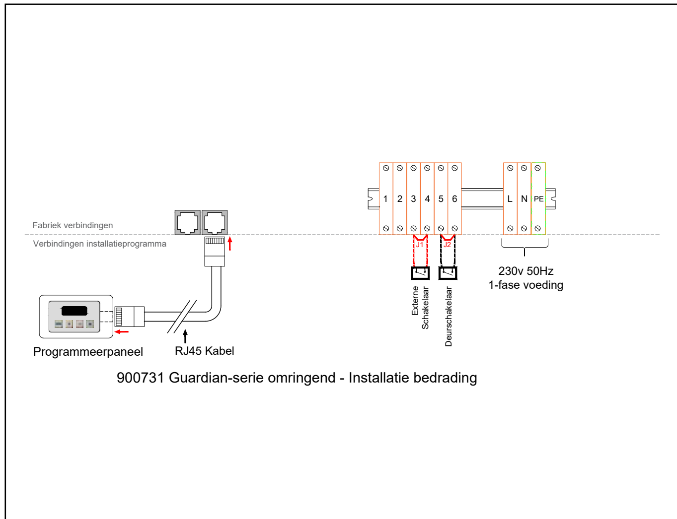
Figuur 20 Bedradingsschema ambient
