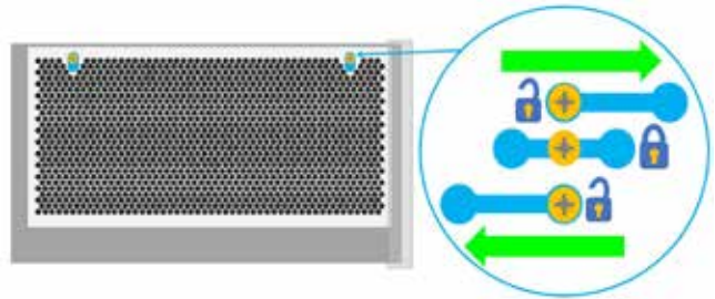
Fig 10 Schroefbevestigingsleuf
