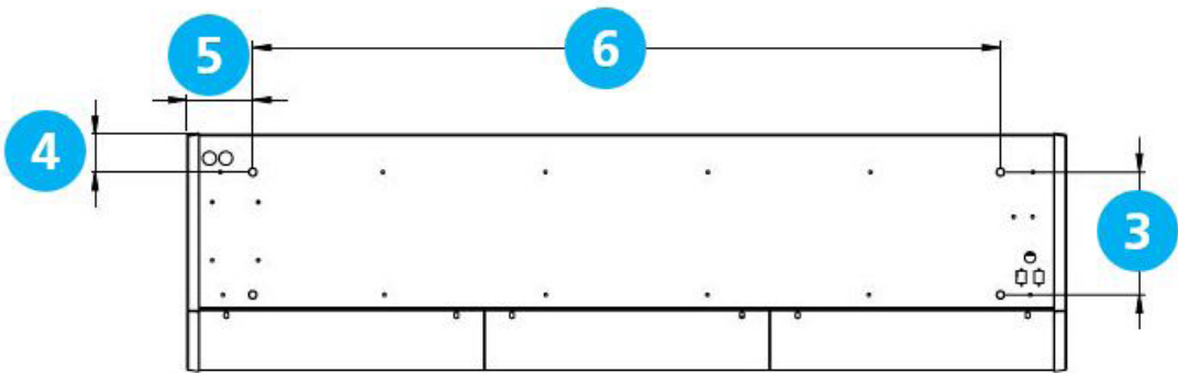
Fig 2 GS Bovenaanzicht
