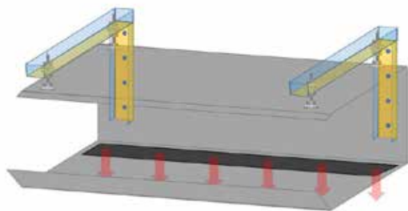
Fig 16 Optie montagebeugel
