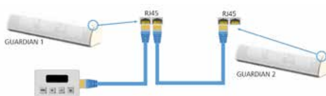
Figuur 25 Bedrading van 2 of meer luchtgordijnen in een netwerk.
