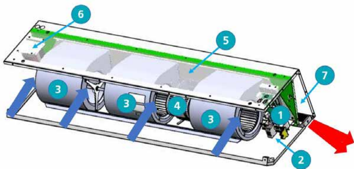
Figuur 6 Componentenindeling GS
