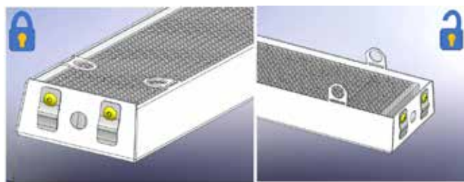
Fig 29 GS-honingraatbevestiging
