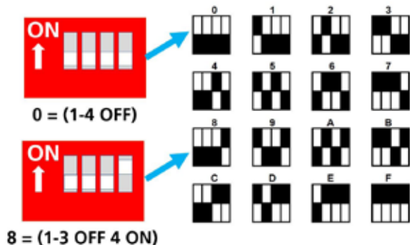
Figuur 24 Luchtgordijn adresnummers
