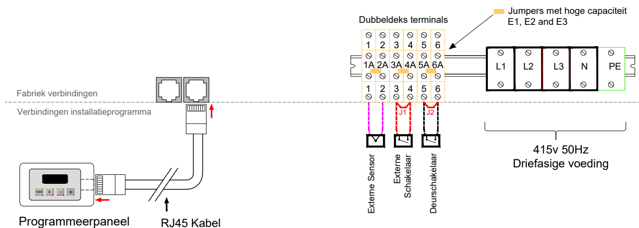
900730 Guardian-serie Elektrisch - Installatie bedrading
