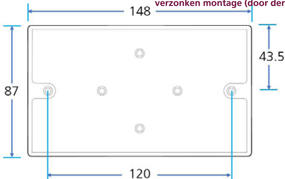
Figuur 5.1 Kunststof doorvoerdoos voor verzonken montage (door derden)
