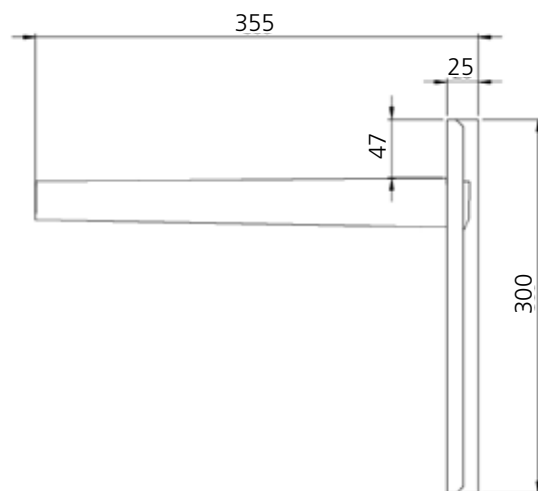
Fig 15.1 Zijaanzicht
