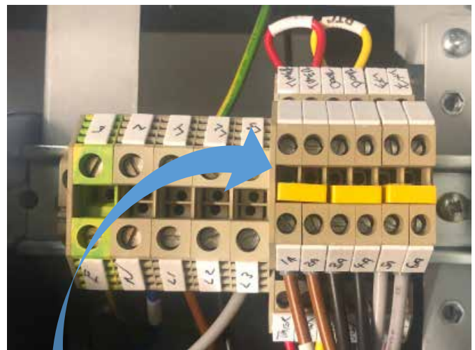
Figure 19.1 Cavaliers de capacité thermique Capacité élevée (cavaliers installés)
