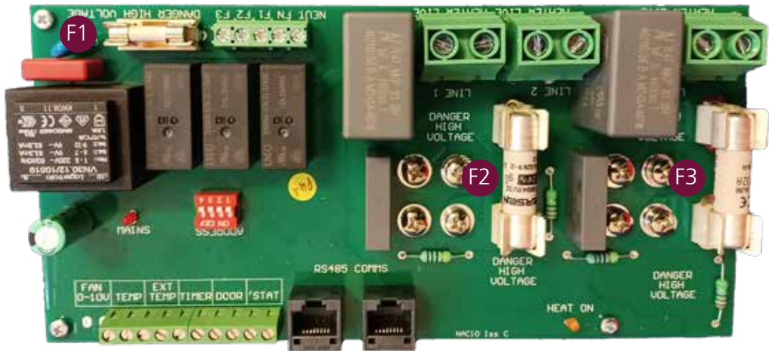
Figure 1 Représentation du modèle électrique de l'emplacement des fusibles
