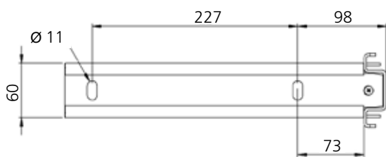
Fig 15.3 Support de montage - vue de dessus
