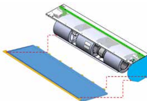
Figure 11 Panneau d'accès inférieur GS
