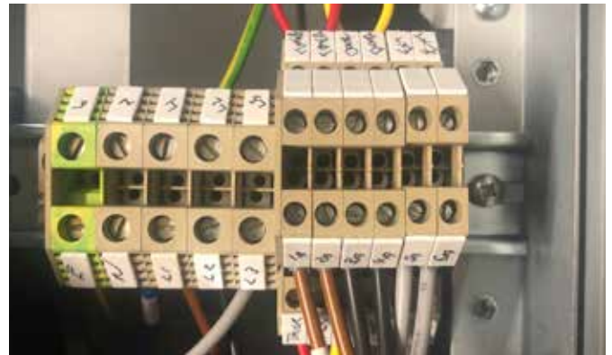
Figure 19 Réglage d'usine des cavaliers de capacité thermique (aucun cavalier installé)
