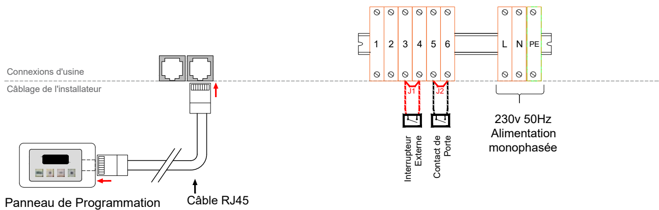
900728 Série Guardian Ambient - Connexions Installateur
