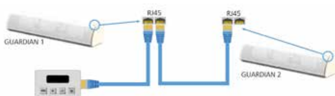
Figure 25 Câblage de 2 ou plusieurs rideaux d'air en réseau.
