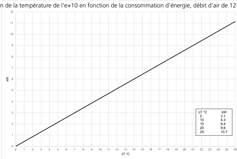
Elévation de la température de l'e+10 en fonction de la consommation d'énergie, débit d'air de 1500m 3 /h (F2)
