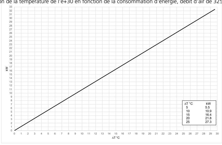
Elévation de la température de l'e+30 en fonction de la consommation d'énergie, débit d'air de 3250m 3 /h (F2)
