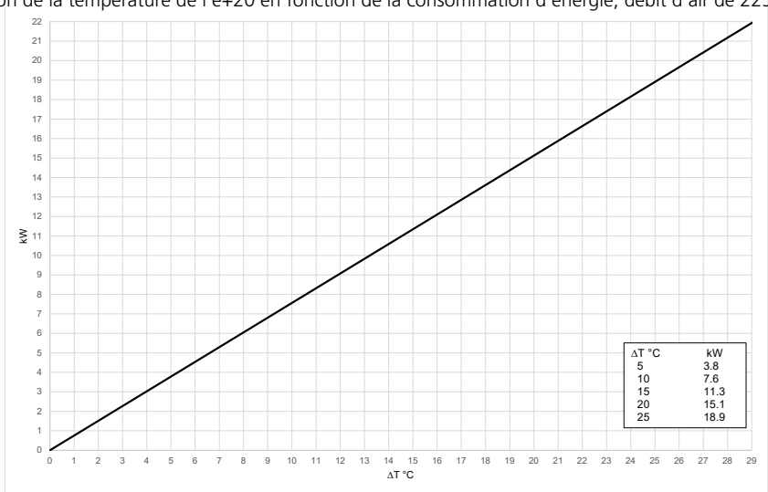
Elévation de la température de l'e+20 en fonction de la consommation d'énergie, débit d'air de 2250m 3 /h (F2)
