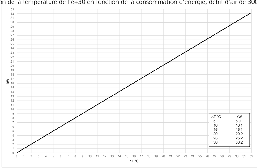
Elévation de la température de l'e+30 en fonction de la consommation d'énergie, débit d'air de 3000m 3 /h (F1)
