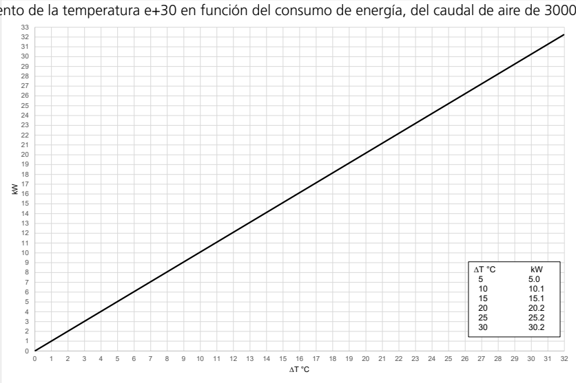
Aumento de la temperatura e+30 en función del consumo de energía, del caudal de aire de 3000m³/h (F1)
