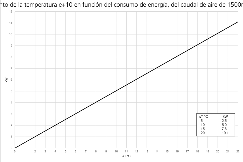
Aumento de la temperatura e+10 en función del consumo de energía, del caudal de aire de 1500m³/h (F2)
