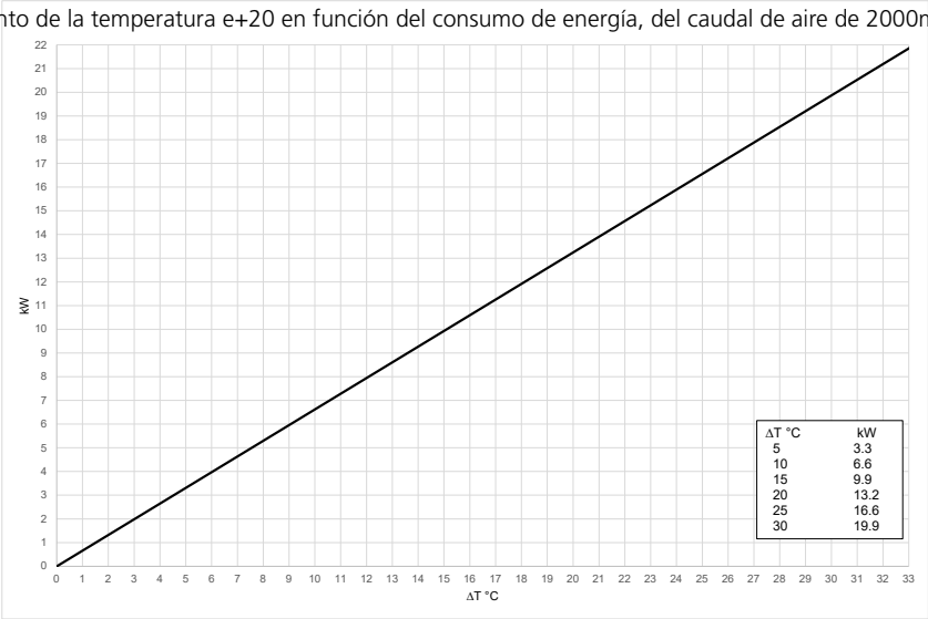
Aumento de la temperatura e+20 en función del consumo de energía, del caudal de aire de 2000m³/h (F1)
