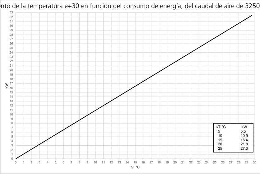
Aumento de la temperatura e+30 en función del consumo de energía, del caudal de aire de 3250m³/h (F2)
