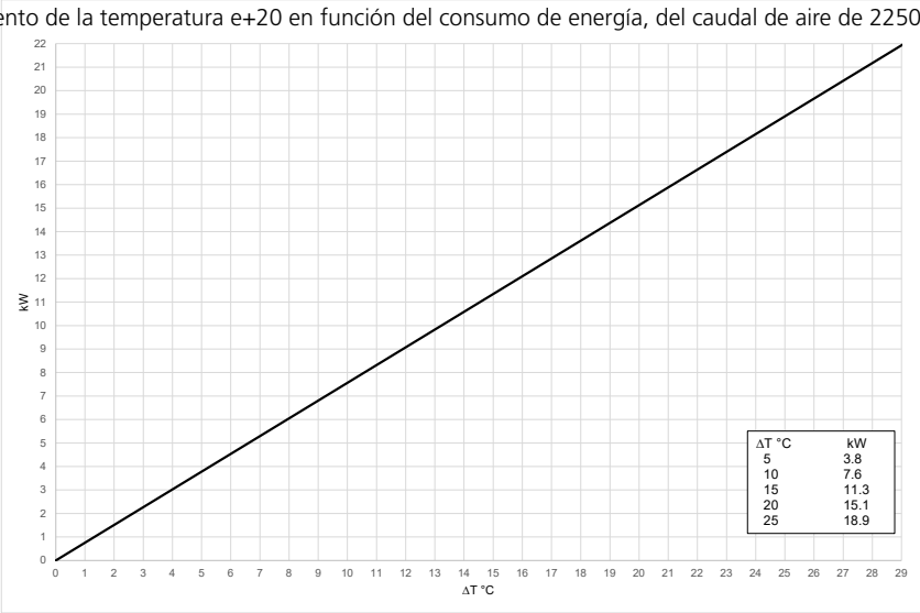
Aumento de la temperatura e+20 en función del consumo de energía, del caudal de aire de 2250m³/h (F2)
