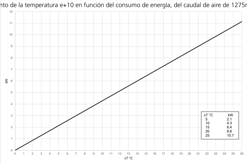
Aumento de la temperatura e+10 en función del consumo de energía, del caudal de aire de 1275m³/h (F1)
