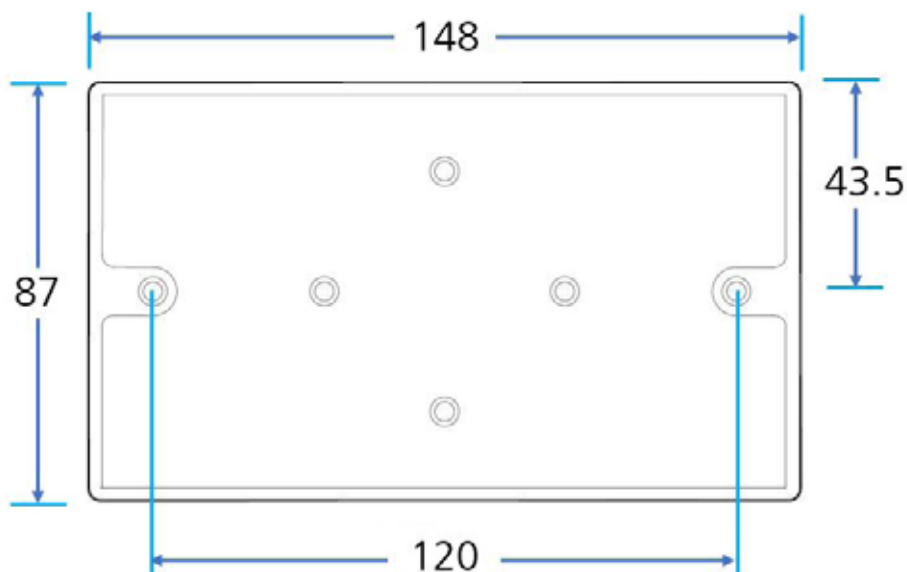
Afbeelding 1.1 Afmetingen opbouwdoos
