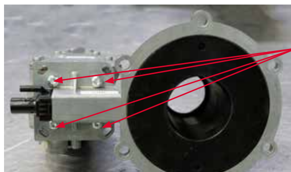
Vis de fixation de la vanne de gaz du Photon 100
