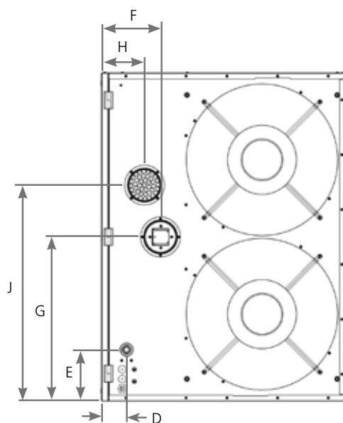
Vue arrière du Photon 120
