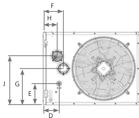
Vue arrière du Photon 10-70
