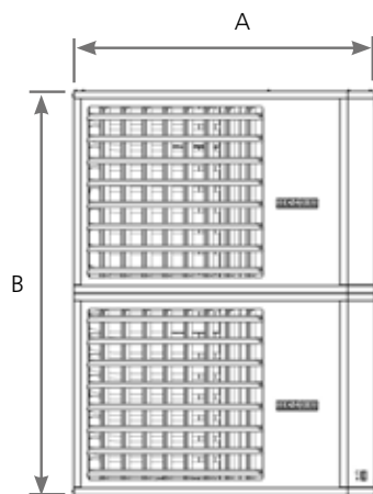
Vue avant du Photon 120
