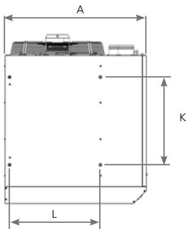
Vue en plan du Photon 10-120
