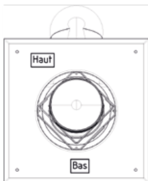
Figure 4a Installation et positionnement ventouse murale
