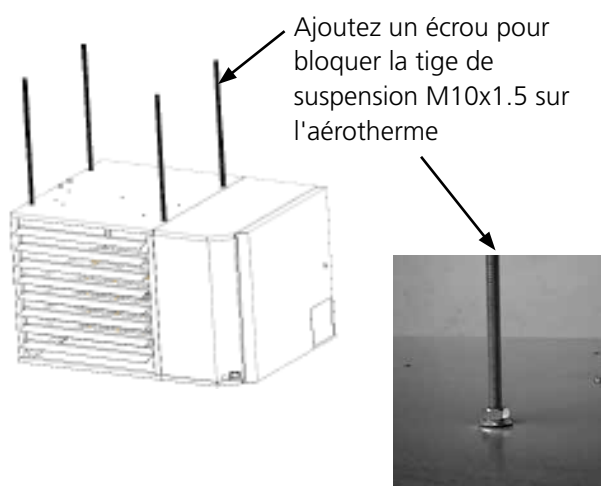
Figure 1 Suspension de l'aérotherme au moyen de tiges à partir des écrous de fixation filetés
