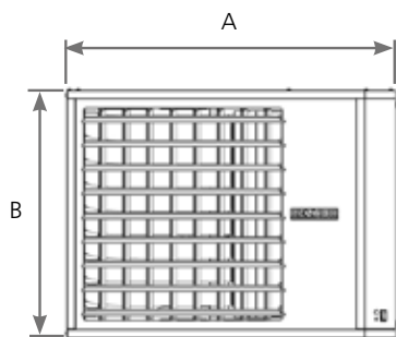
Vue avant du Photon 10-100
