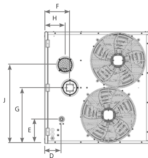
Vue arrière du Photon 100
