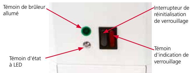
Interrupteur de réinitialisation et témoins d'état
