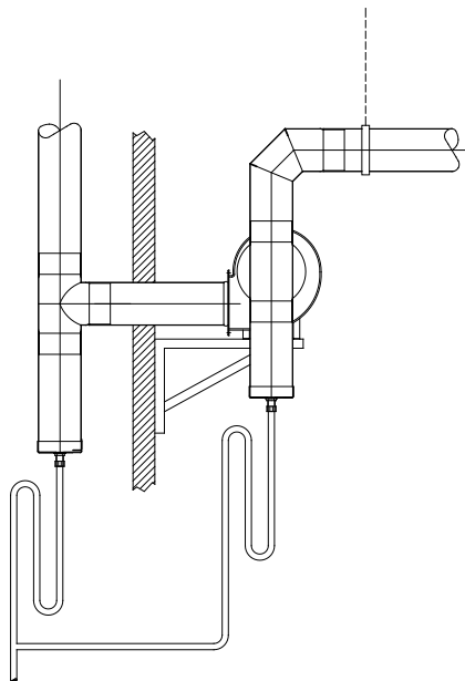
Ilustración 6.5 Salida de pared para disposición de salida de humos convencional
