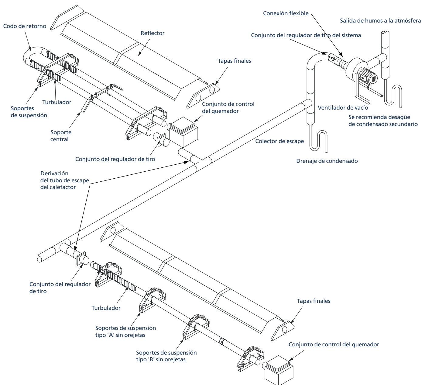
Ilustración 8. Instalación en espiga
