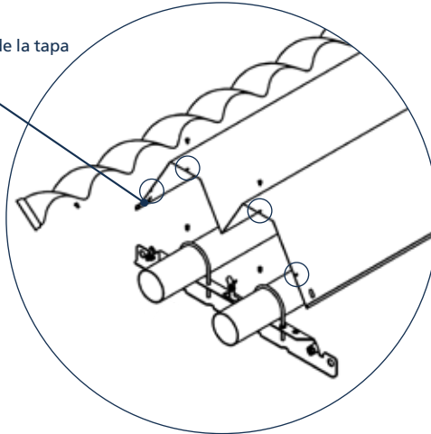
Ilustración 29. Reflector en V de tubo en U final
