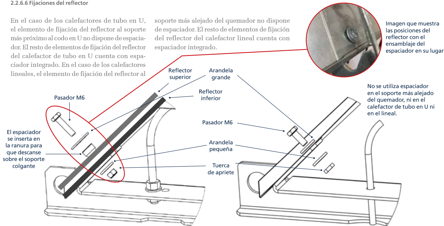
Ilustración 31. Reflector en V de tubo en U intermedio
