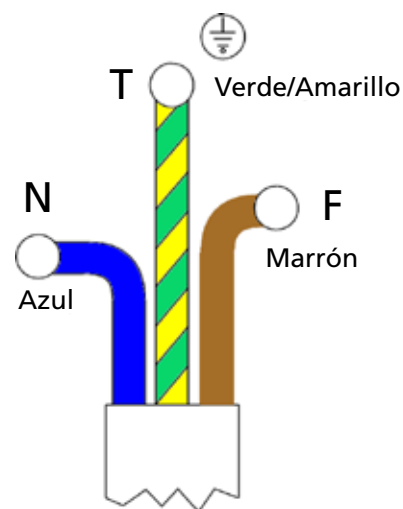
Ilustración 14. Cableado monofásico
