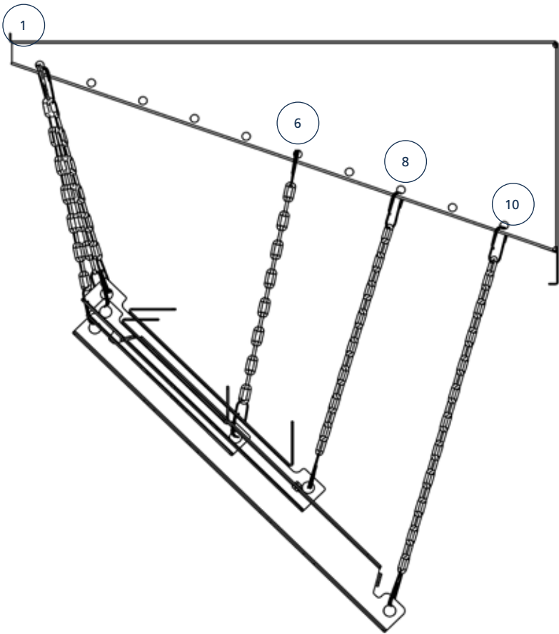
Ilustración 1. Montaje en ángulo utilizando el soporte de montaje en pared
