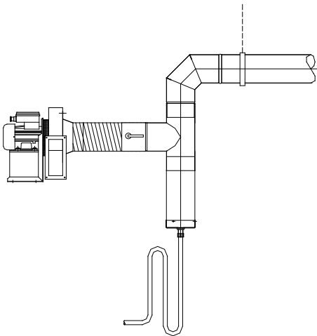
Ilustración 6.7 Disposición típica de ventilador bajo
