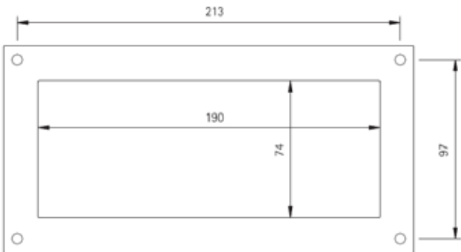
Ilustración 6.2 Dimensiones de la salida del ventilador tipo '0'
