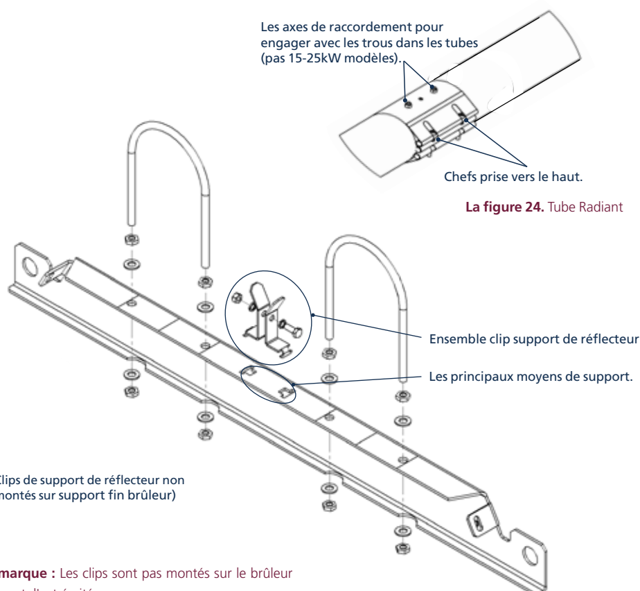
La figure 25. Support de réflecteur
