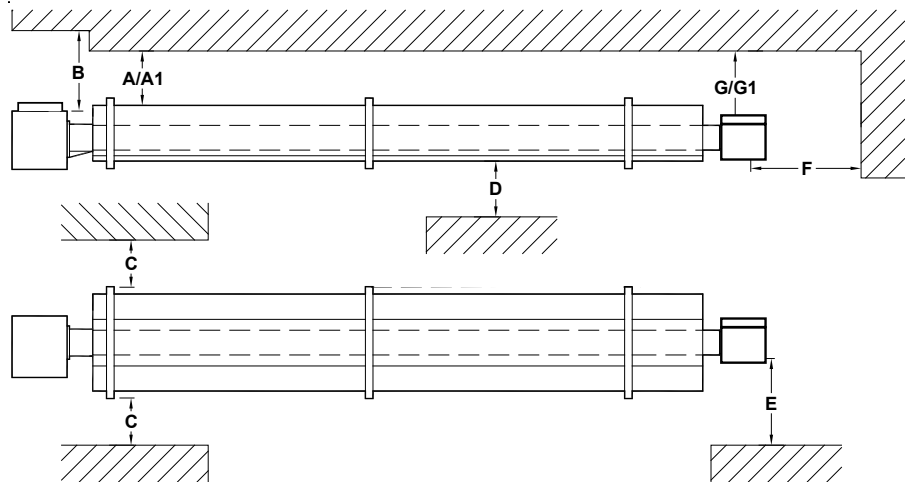
Figure 10. Diagrama que ilustra a folga para combustíveis (Linear mostrado)
