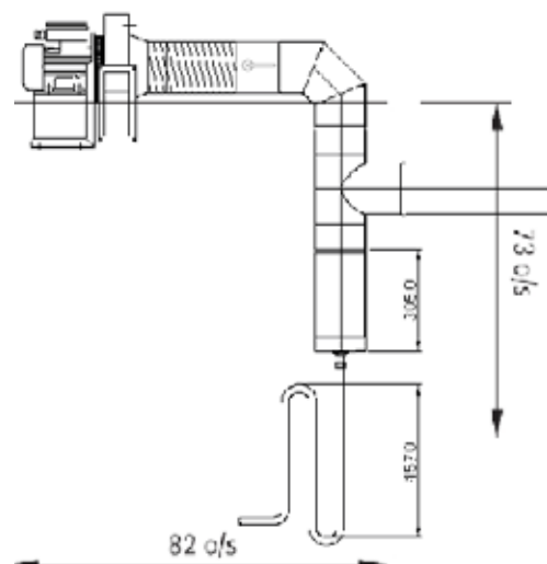
Figuur 6.3 Type 2 ventilatoruitgang afmetingen
