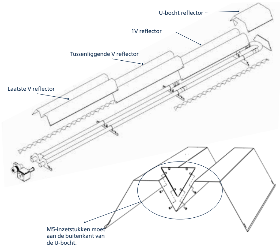
Figuur 28. Reflectoren
