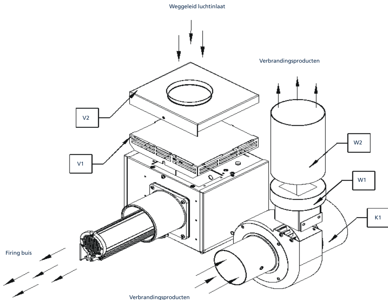
Figuur 18. Optie 1. Flue Attachment geïnduceerde branders (VSUTE)
