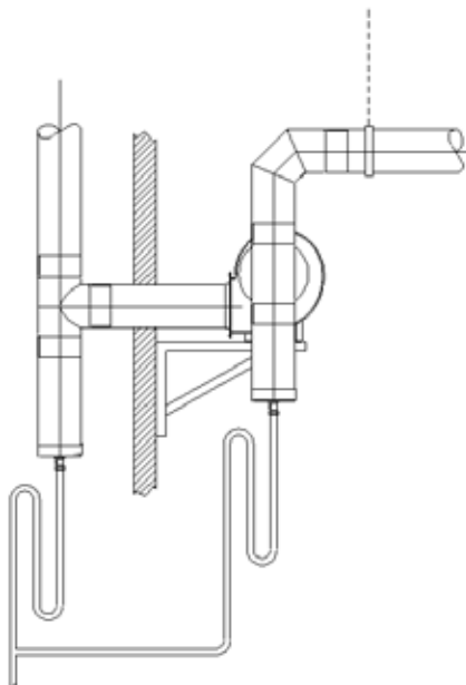
Figuur 6.5 Conventionele flue regeling muur uitgang
