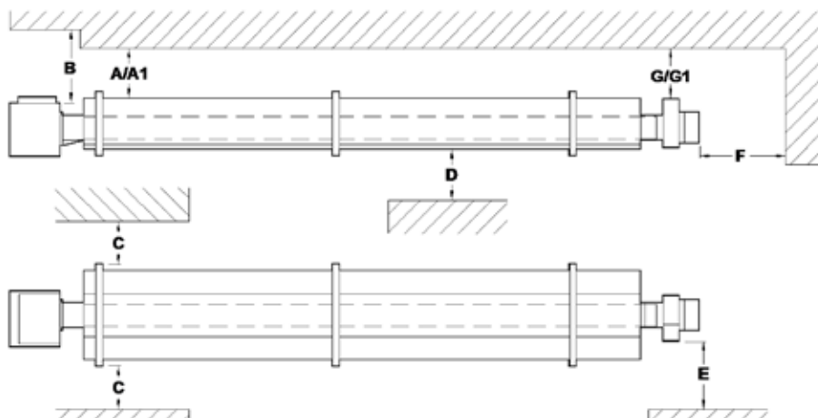
Figuur 9. Diagram waarin de afstand tot brandbare stoffen (U-buis weergegeven)
