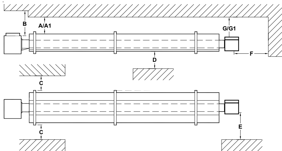
Figure 10. Esquema que ilustra la distancia a los combustibles (lineal)
