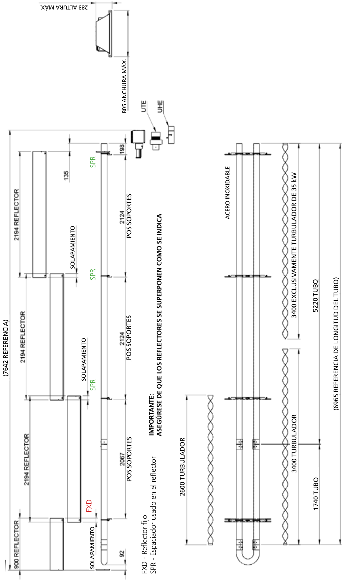
Figure 43. Conjunto del calefactor Vision: Modelos VSUTE/SUHE 35 kW. Diá. nom. 100 mm (4 pulg)
