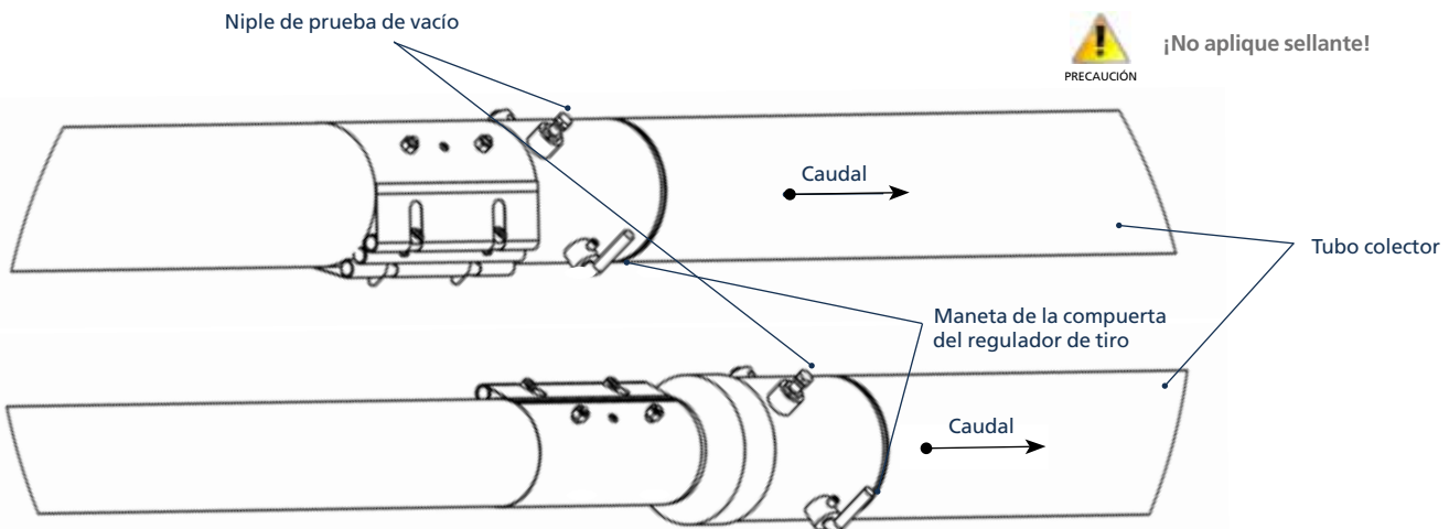
Figure 39.1 Conjunto del regulador de tiro en espiga
