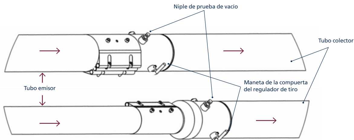
Figure 51. Conjunto del regulador de tiro en espiga
