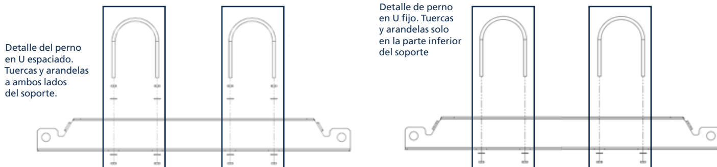
Figure 26.2 Fijación de pernos en U en los soportes de suspensión del calefactor de tubo en U
