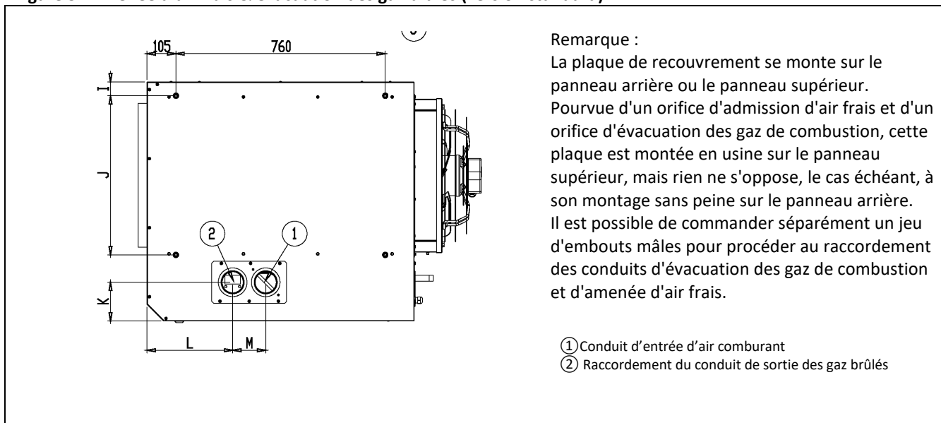
Figure 5 : Aménée d'air frais & évacuation des gaz brûlés (version standard)
