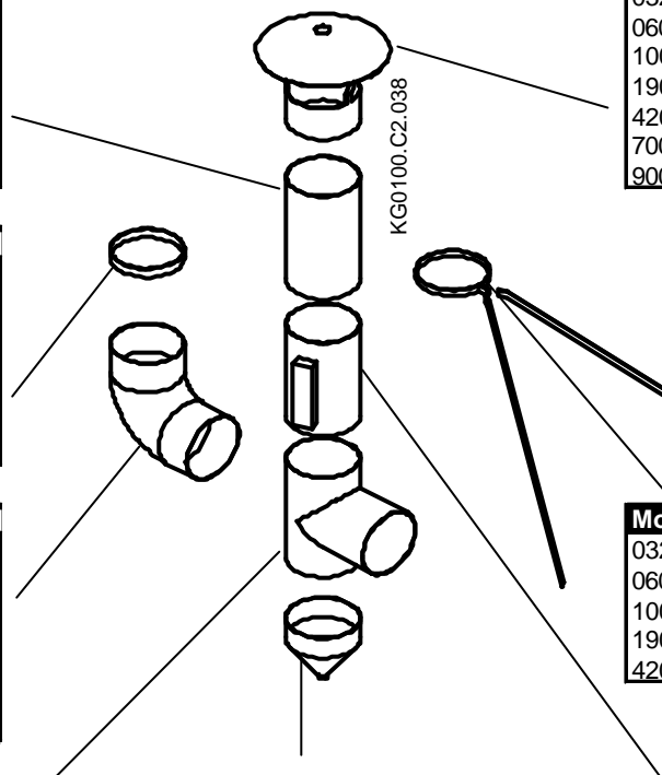
Condensate collector
