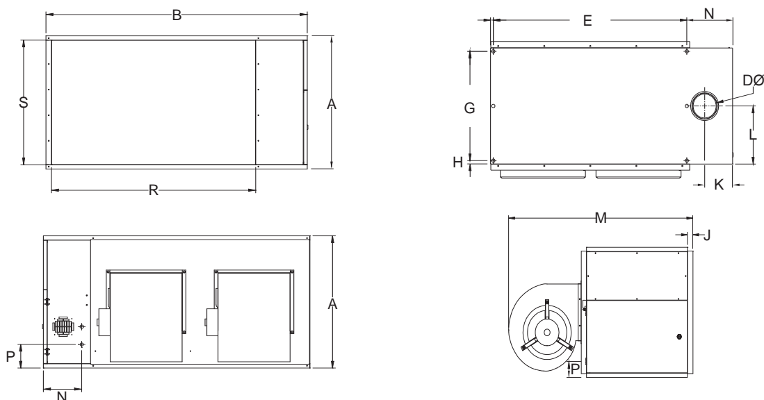
OUHC Centrifugal Fan
