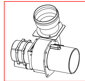
Bloc extracteur
